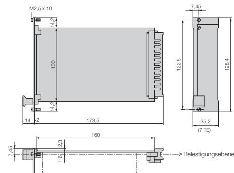
Bild 2. Frontplattenbreite 7 TE.
